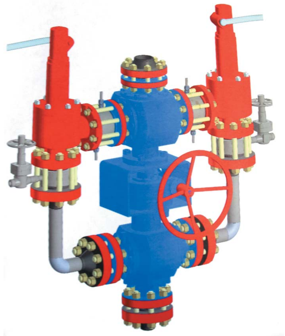
Блок синхронного переключения пружинно-предохранительных клапанов
