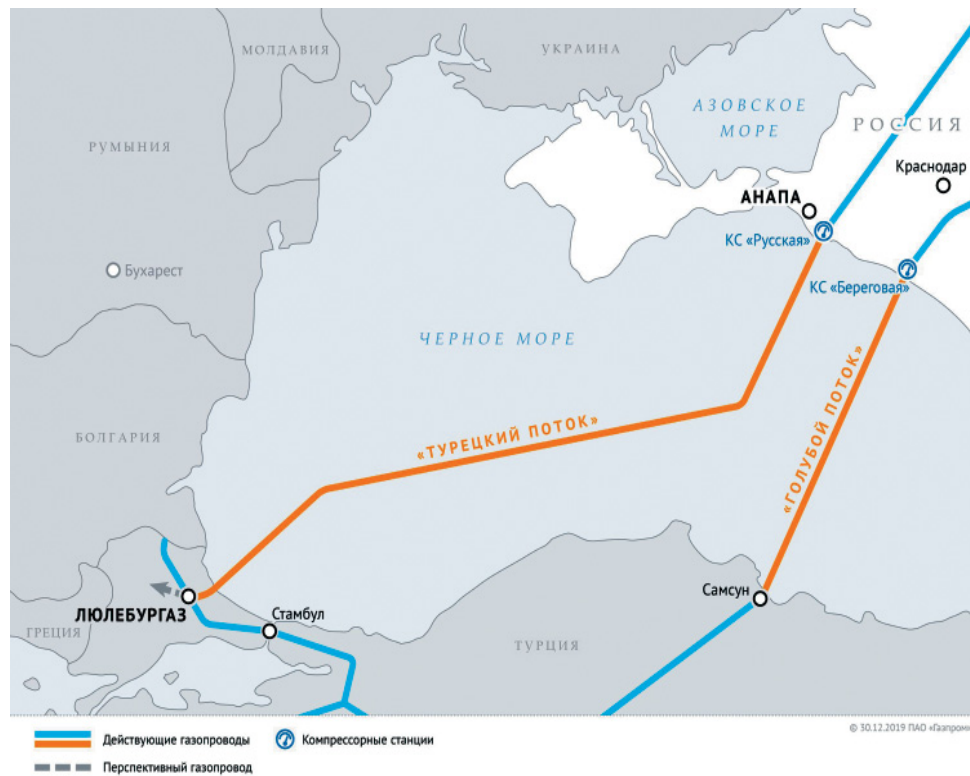
■ Схема газопроводов «Турецкий поток» и «Голубой поток»
